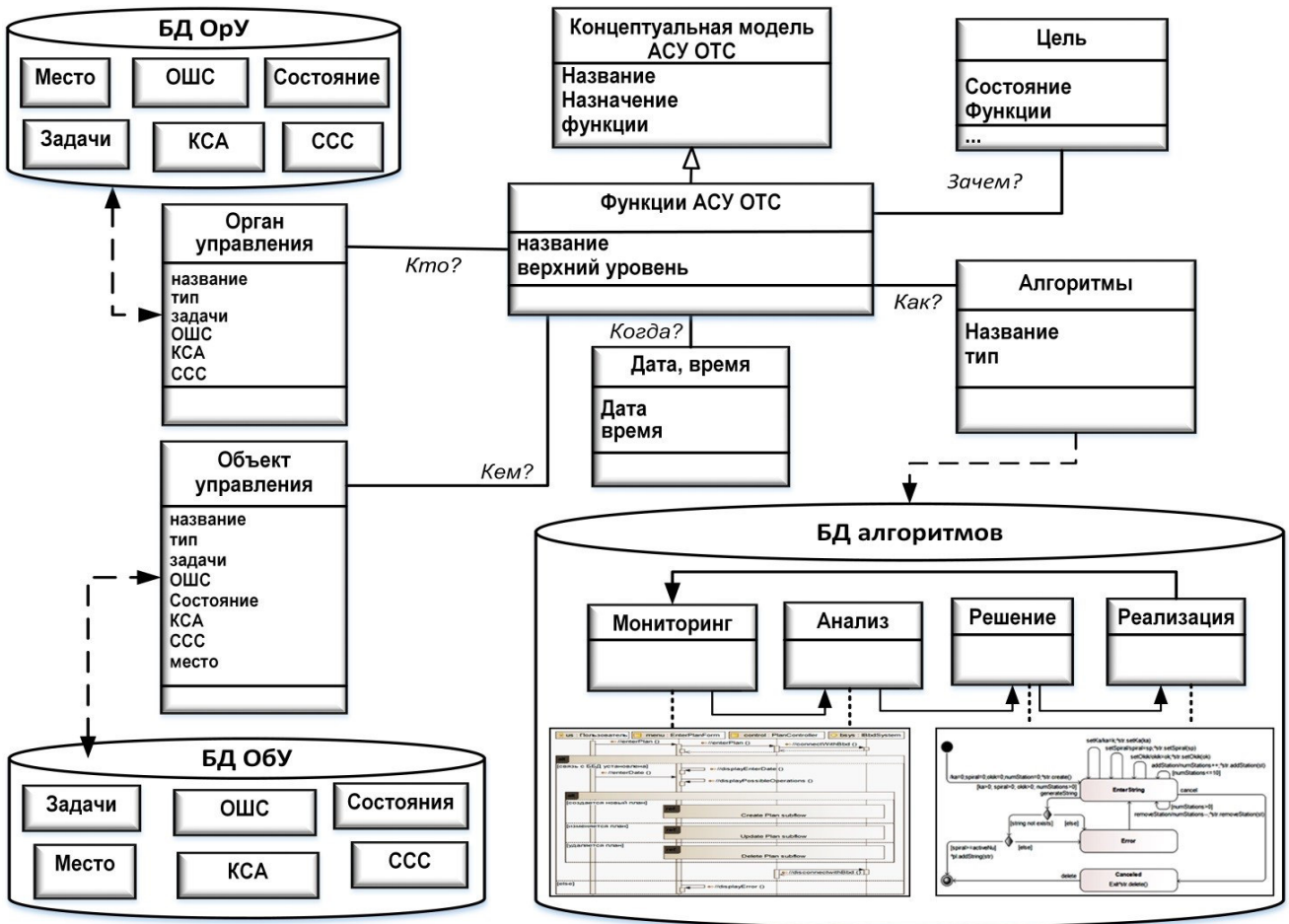
Рис. 4. Расширенная концептуальная модель АСУ ОТС
