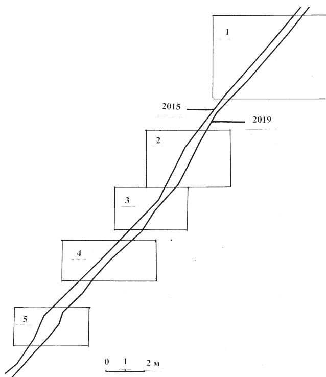
Рис. 2. Фрагмент профиля осыпного склона, сложенного алевролитами. Цифрами в прямоугольниках обозначены участки склона с различной крутизной.
