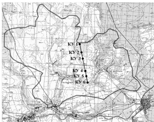
Рис. 1. Водосборный бассейн р. Майдан и объекты исследования.
