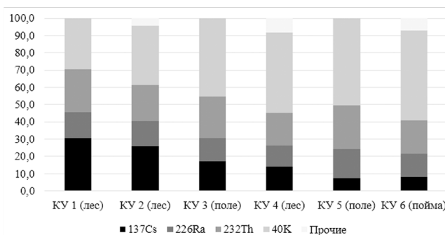
Рис. 2 Вклад почвенных радионуклидов в формирование мощности дозы гамма-излучения (в %).
