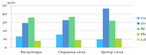
Рис. 2. Содержание тяжелых металлов в почвах района исследований.
