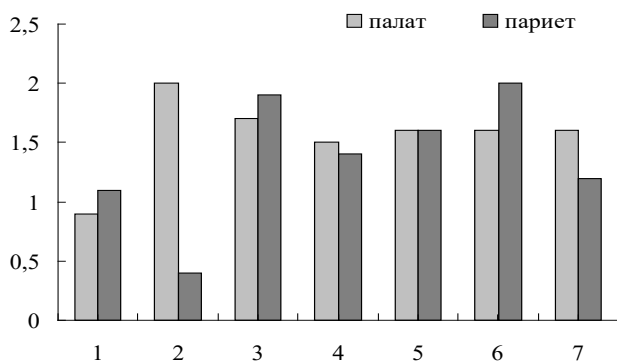
Рис. 5. Параметры средних значений развития устьевых зубов (палатального и париетального) раковины Ch. tridens . Обозначения см. рис. 1.
