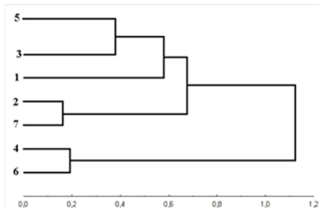
Рис. 3. Дендрограмма сходства популяций Ch. tridens по основным параметрам (BP, ШР, ВУ, ШУ) раковины. Обозначения см. рис.1.
