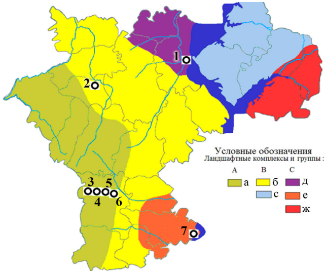
Рис. 1. Расположение точек сбора популяций моллюсков в выделенных типах ландшафтов Ульяновской области (Артемьева, др., 2018). 1 – г. Ульяновск (54,31° с.ш. и 48,40° в.д.), 2 – окрестности с. Бекетовка Вешкаймского района (54,06° с.ш. и 46, 52° в.д.), 3 – окрестности с. Давыдовка Николаевского района (53,06° с.ш. и 47,16° в.д.), 4 – окрестности с. Прасковьино (Шихан-гора) Николаевского района (53,04° с.ш. и 47,15° в.д.), 5 – окрестности с. Акуловка (р. Ардовать) Николаевского района (53,04° с.ш. и 47,25° в.д.), 6 – окрестности с. Варваровка Николаевского района (53,05° с.ш. и 47,48° в.д.), 7 – окрестности с. Вязовка Радищевского района (52,52° с.ш. и 48,22° в.д.).
