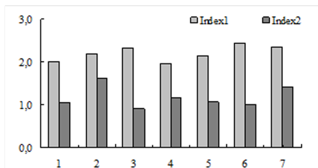
Рис. 4. Параметры средних значений индексов устья раковины Ch. tridens . Обозначения см. рис.1.
