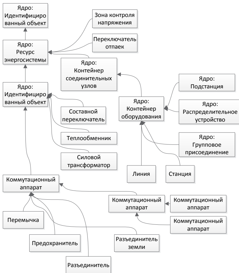
Рис. 3. Классификация оборудования по IEC 61970-301
