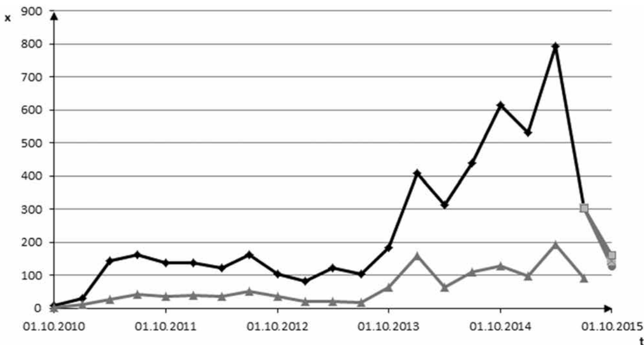
Рис. Прогнозирование появления ошибок в проекте «FreeNAS9» с учетом влияния добавления новых функциональных возможностей в проект (гипотеза прогноза на заданный период)
