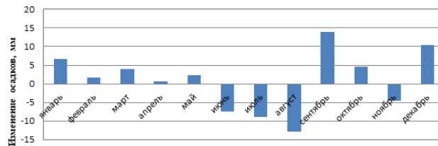
Рис. 6. Внутригодовое изменение осадков по территории Ульяновской области за 1961 – 2018 гг.
