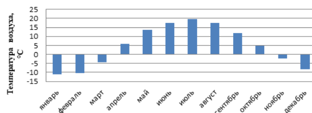
Рис. 1. Годовой ход температуры воздуха за 1961 – 2018 гг.
