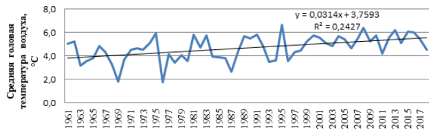
Рис. 2. Динамика средней годовой температуры воздуха за 1961–2018 гг.
