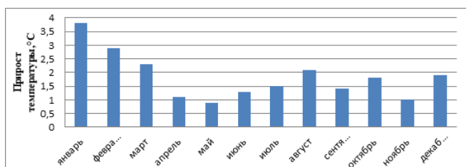
Рис. 3. Внутригодовое распределение прироста температуры осредненного по территории Ульяновской области за 1961–2018 гг.
