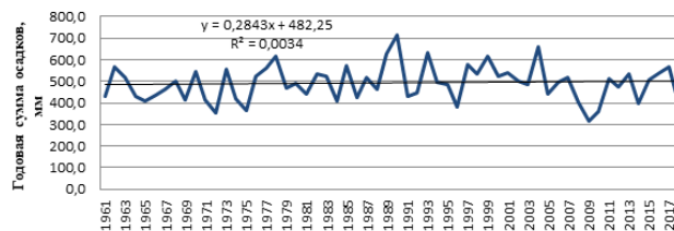
Рис. 5. Межгодовая изменчивость сумм осадков за период 1961–2018 гг.
