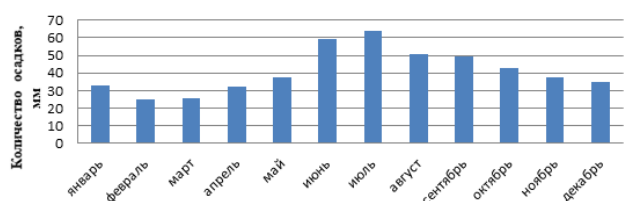
Рис. 4. Внутригодовое распределение осадков на территории Улья-
