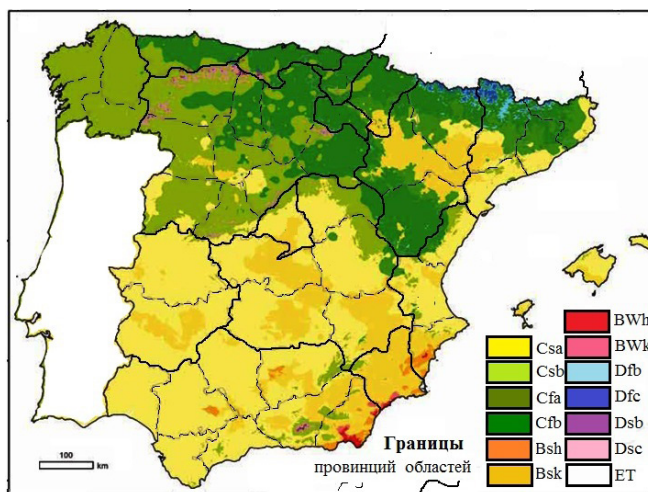
Рис. 1. Типы климата Испании согласно климатической классификации Кёппена – Гейгера.
